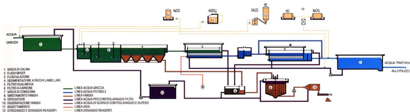
QUADRO DI CONTROLLO SOLLEVAMENTO E POTABILIZZATORE ACQUE DEL FIUME IMERA (CALTANISSETTA-ITALIA) CONTROL BOARD FOR THE WATER PUMPAGE AND TREATMENT PLANT OF IMERA RIVER (CALTANISSETTA-ITALY)
