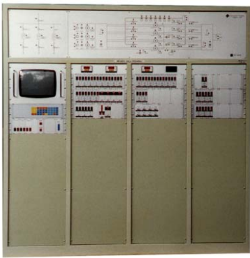
QUADRO DI CONTROLLO IMPIANTO DI SOLLEVAMENTO SUL FIUME PO ISOLA PESCAROLI (MANTOVA-ITALIA) CONTROL BOARD FOR THE WATER PUMPAGE PLANT ON PO RIVER ISOLA PESCAROLI (MANTOVA-ITALY)
