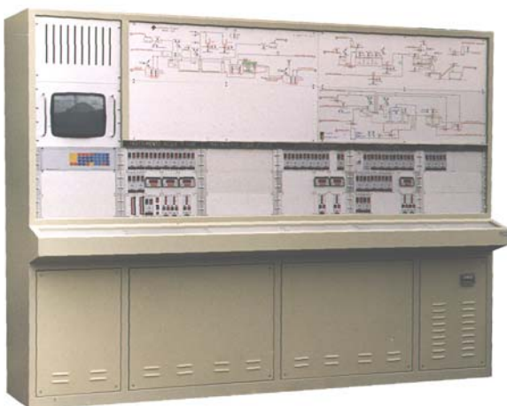
QUADRO DI CONTROLLO PER DEPURATORE INDUSTRIALE SOC. BOSELLI s.p.a. (COMO-ITALIA) CONTROL BOARD FOR THE INDUSTRIAL PURIFICATION PLANTS OF BOSELLI s.p.a. (COMO-ITALY)
